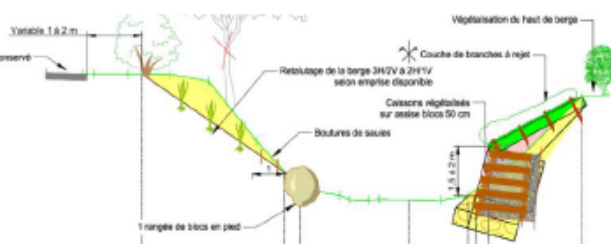
Schéma des protections des berges en aval de la passerelle de l'ancienne scierie
