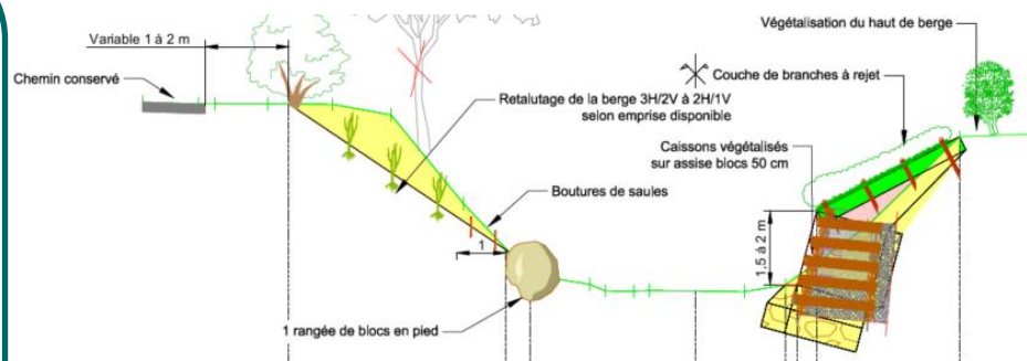
Schéma des protections des berges en aval de la passerelle de l'ancienne scierie
