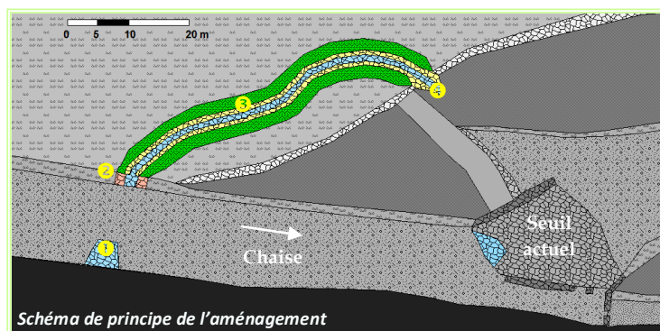
Prise d'eau amont
